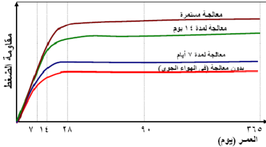
تأثير المعالجة على مقاومة الخرسانة.
